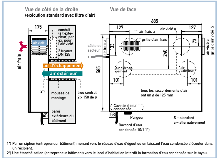
Fig. 1 : Dimensions
