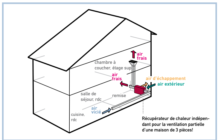
Fig. 2 : Solution d'îlot pour ventilation partielle avec de courts conduits
